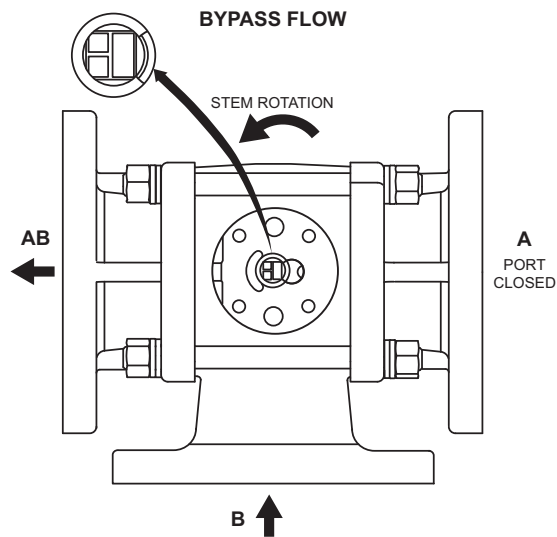
Fig. 11. Stem Rotation
