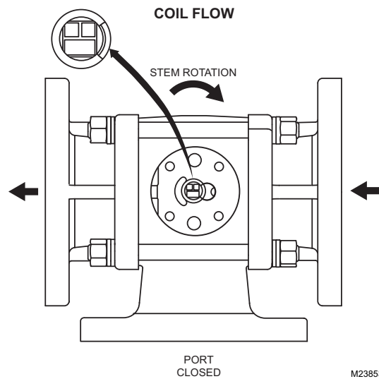
Fig. 11. Stem Rotation
